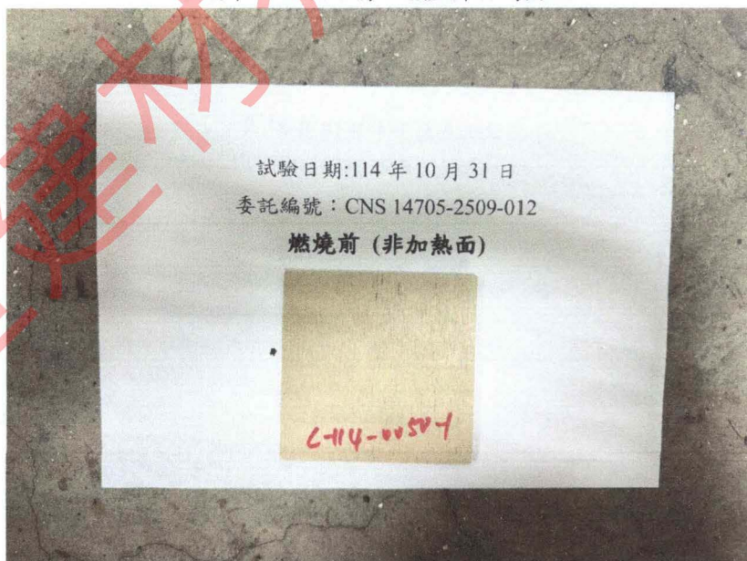
照片 2 試驗前試體非加熱面
