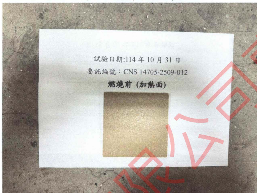
照片 1 試驗前試體加熱面
